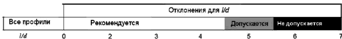
Рисунок 13 - Рекомендации по выбору оптимального соотношения длины пути утечки к межреберному расстоянию
