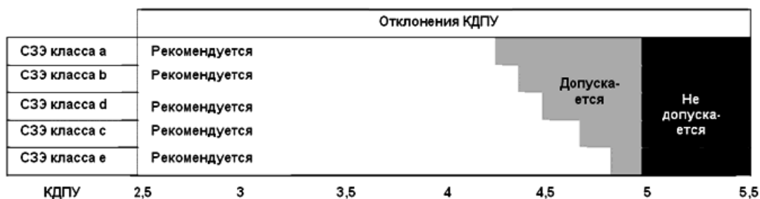
Рисунок 16 - Рекомендации по выбору коэффициента длины пути утечки
