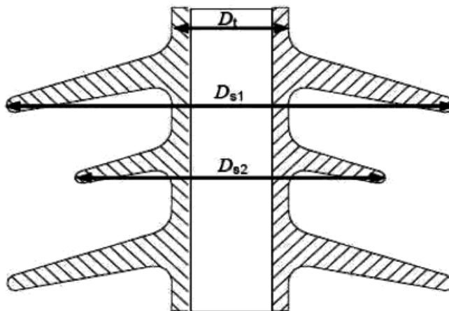
Рисунок 17а - Иллюстрация параметров D_t , D_{s1} и D_{s2}
