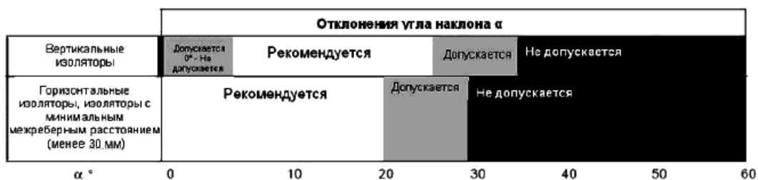
Рисунок 15 - Рекомендации по выбору угла наклона ребра
