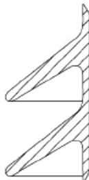
Рисунок 3 - Типичный профиль с крутым наклоном ребра
