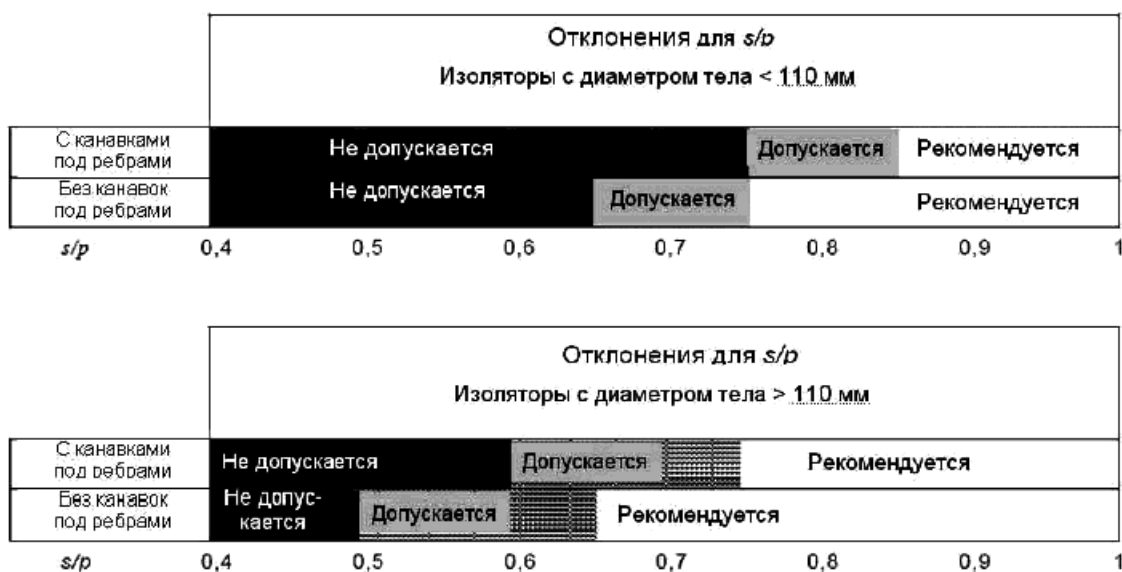
Рисунок 8 - Межреберное расстояние для разных профилей изоляторов
