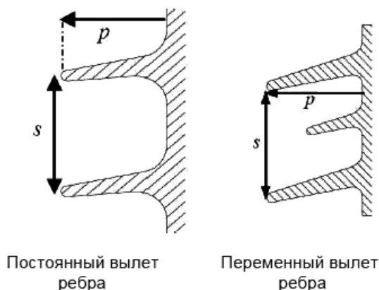
Рисунок 8 - Межреберное расстояние для разных профилей изоляторов
