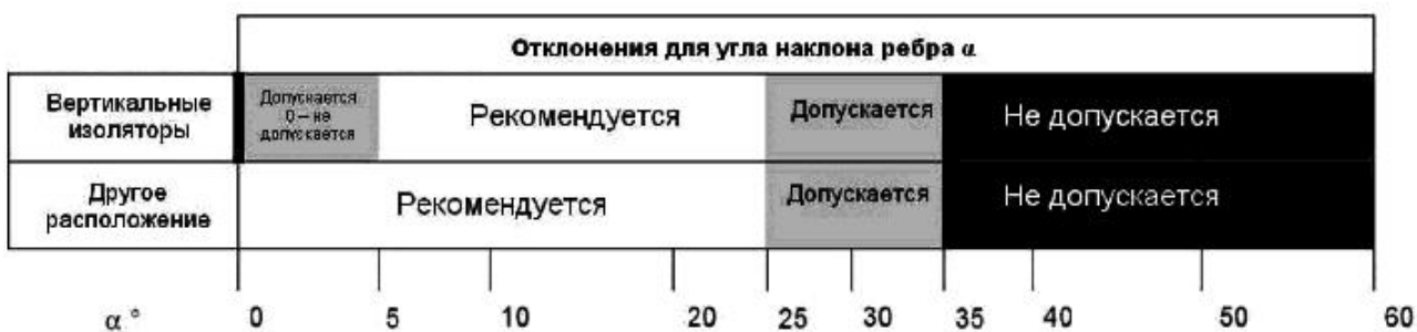
Рисунок 14б - Рекомендации по выбору угла наклона ребра
