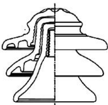
Рисунок 6б - Многослойный штыревой изолятор
