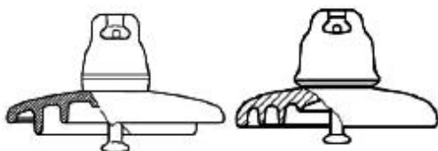
Рисунок 2а - Стандартные тарельчатые изоляторы
