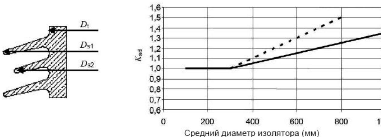
Рисунок 16 - K_{ad} в зависимости от диаметра изолятора
