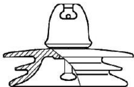
Рисунок 5а - Тарельчатые изоляторы с переменным вылетом ребра
