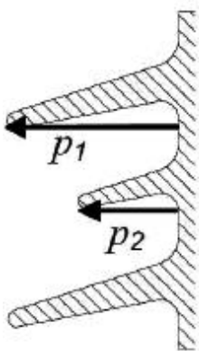
Рисунок 7 - Переменный профиль ребер
