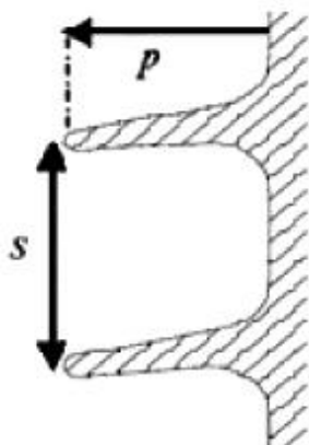
Рисунок 8а - Постоянный вылет ребер
