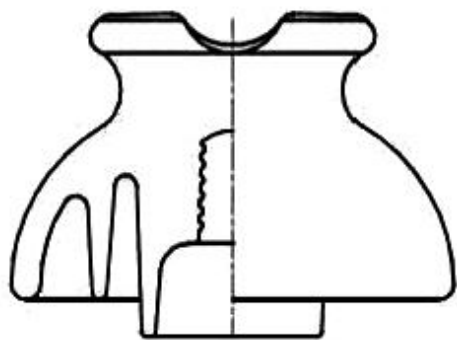
Рисунок 6а - Цельный штыревой изолятор
