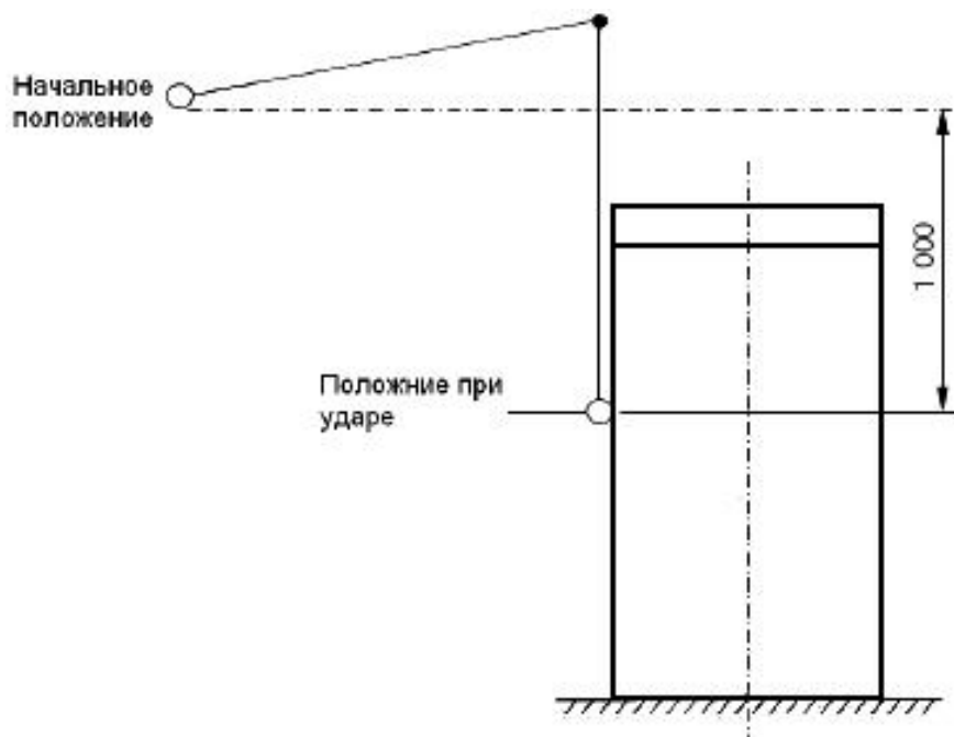
Рисунок 103б - Схема проведения испытания для подтверждения стойкости к удару при монтаже НКУ-ОП-Д на земле без фиксации в основании
