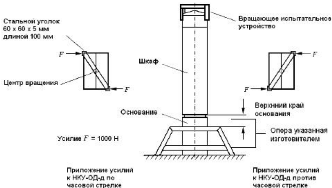
Рисунок 106а - Схема проведения испытания для подтверждения стойкости к скручиванию при монтаже НКУ-ОП-Д на земле, зафиксированного в предназначенном состоянии
