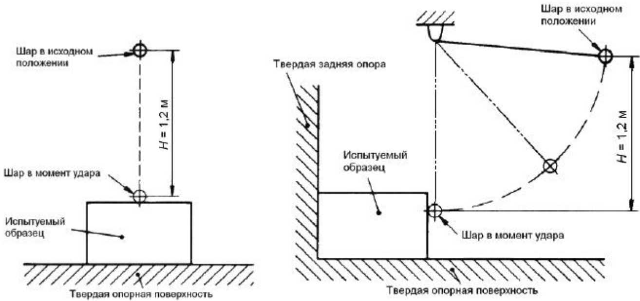
Рисунок 101 - Испытания на удар с помощью стального шара
