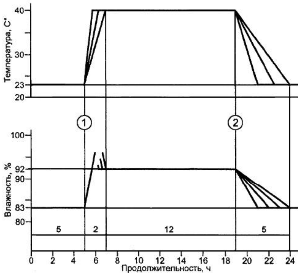
Рисунок 102 - График температуры и влажности
