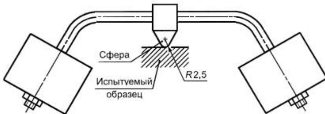
Рисунок 1 -Установка для испытания на теплостойкость
