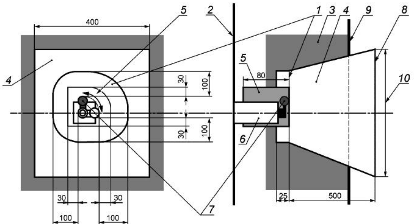
Рисунок 4 - Рабочее пространство для оперирования поворотными устройствами
