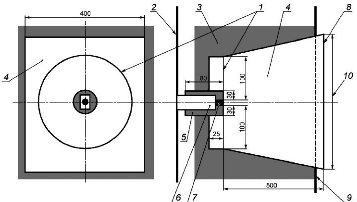
Рисунок 3 - Рабочее пространство для оперирования кнопками
