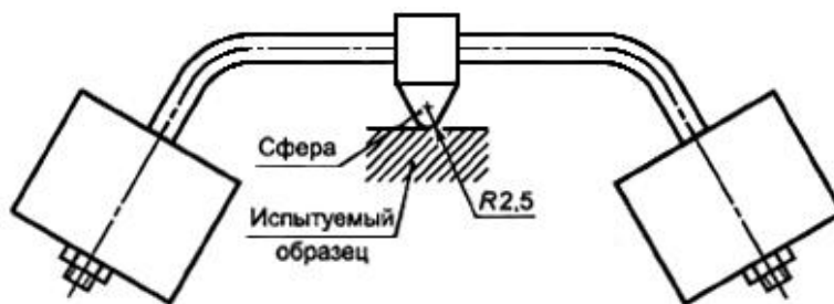
Рисунок 1 - Установка для испытания на теплостойкость
